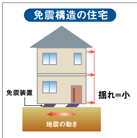
免震構造の住宅と一般の住宅の違い
