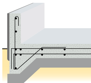
鉄筋コンクリート造のべた基礎
